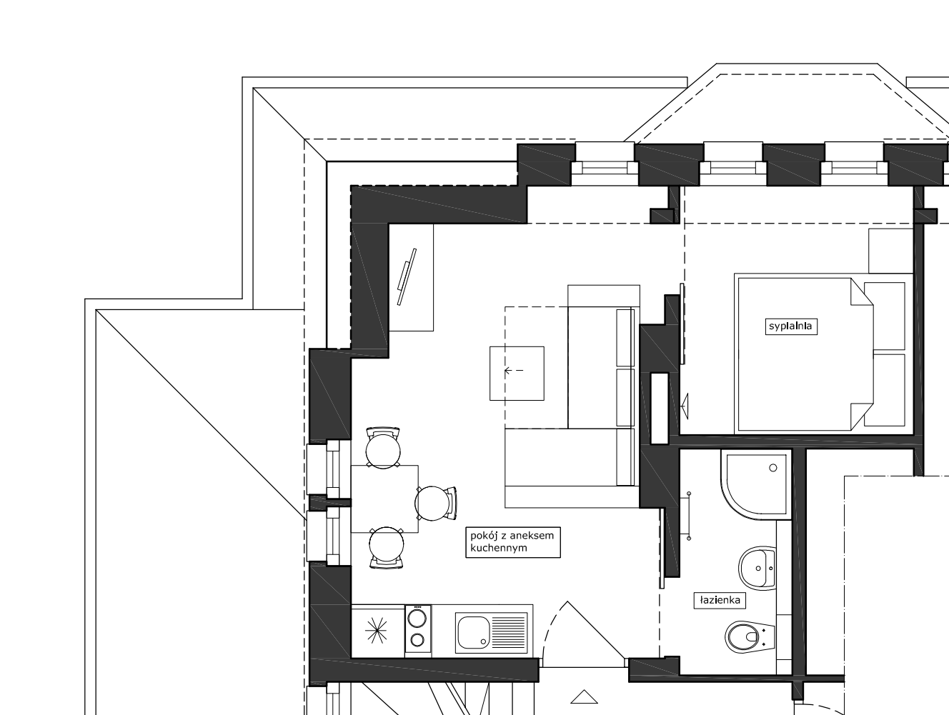
PLAN APARTAMENTU
