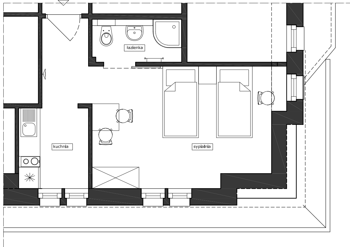
PLAN APARTAMENTU
